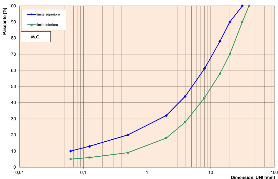
DIAGRAMMA GRANULOMETRICO
